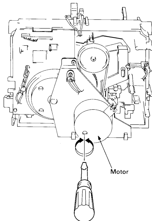
Fig. 11-2 Diagrama de disposición de las partes de ajuste
