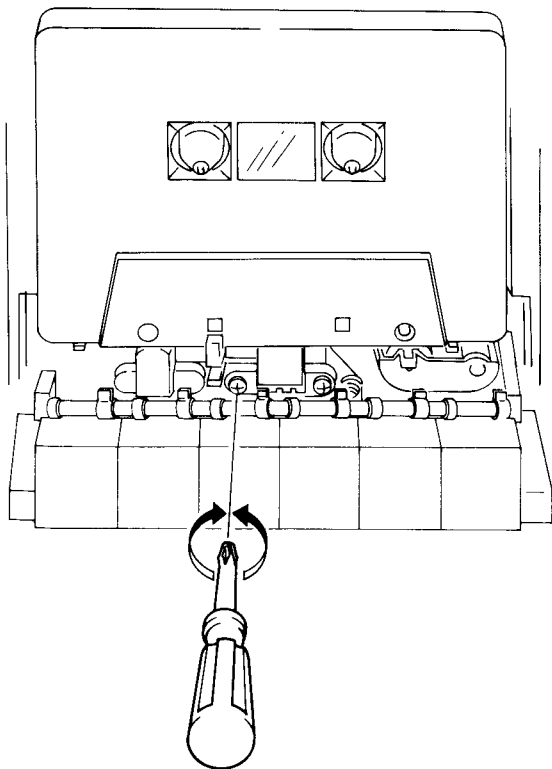
Fig. 11-5 Réglage d'azimut de la tête
